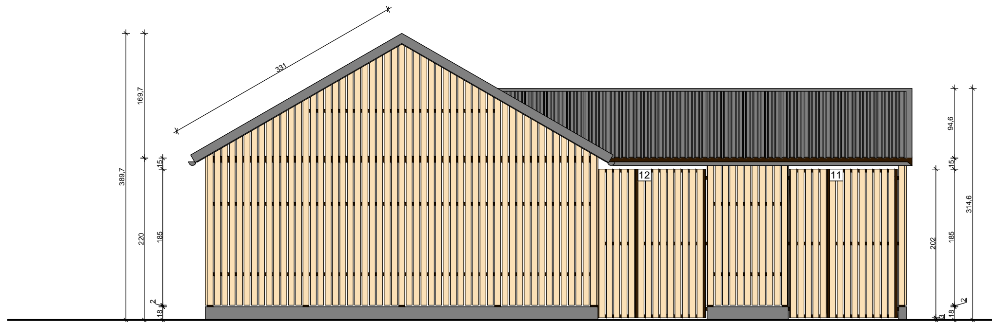
ELEWACJA PÓLNO-CNO-WSCHODNIA
